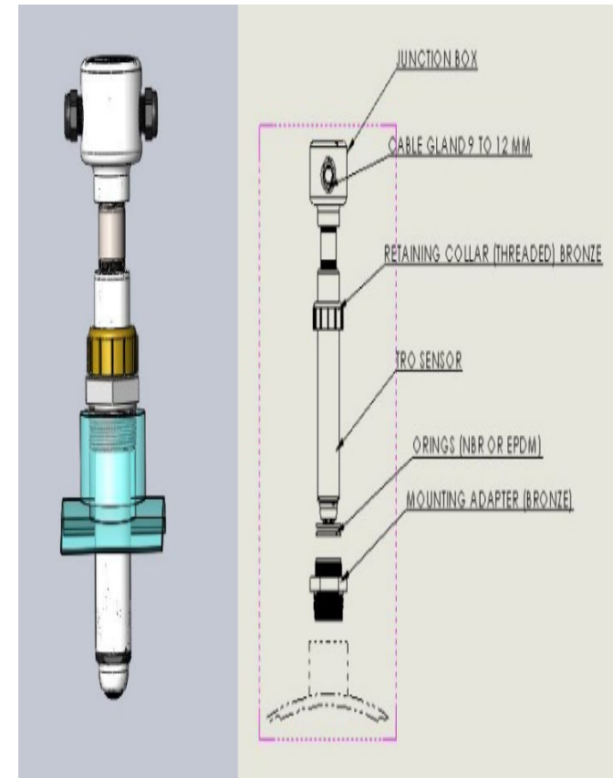
T.R.O Analyzer
