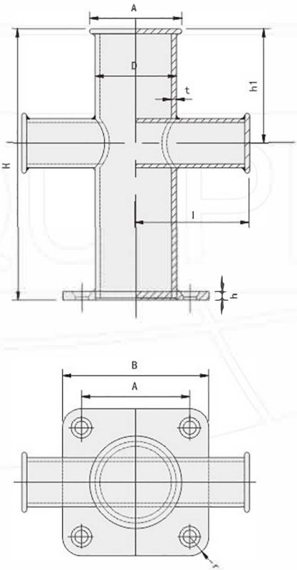
D型 - 带缆桩 Model D Bollard Bitt
