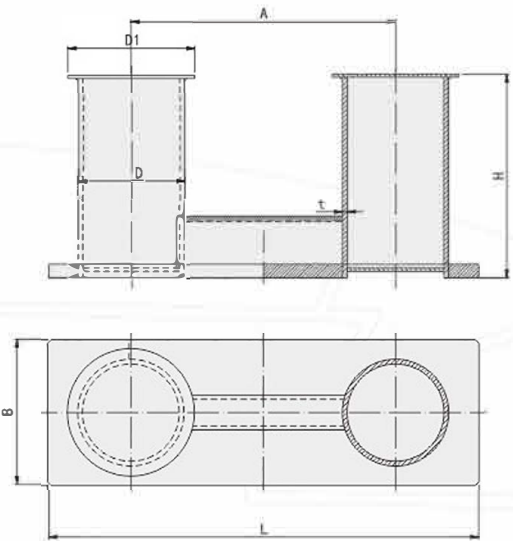
C型 - 带缆桩 Model C Bollard Bitt
