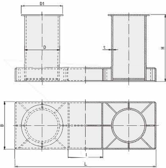
A、B型参数 Parameters of Model A and Model B
