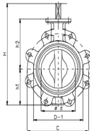
Lug type.....Series 52
